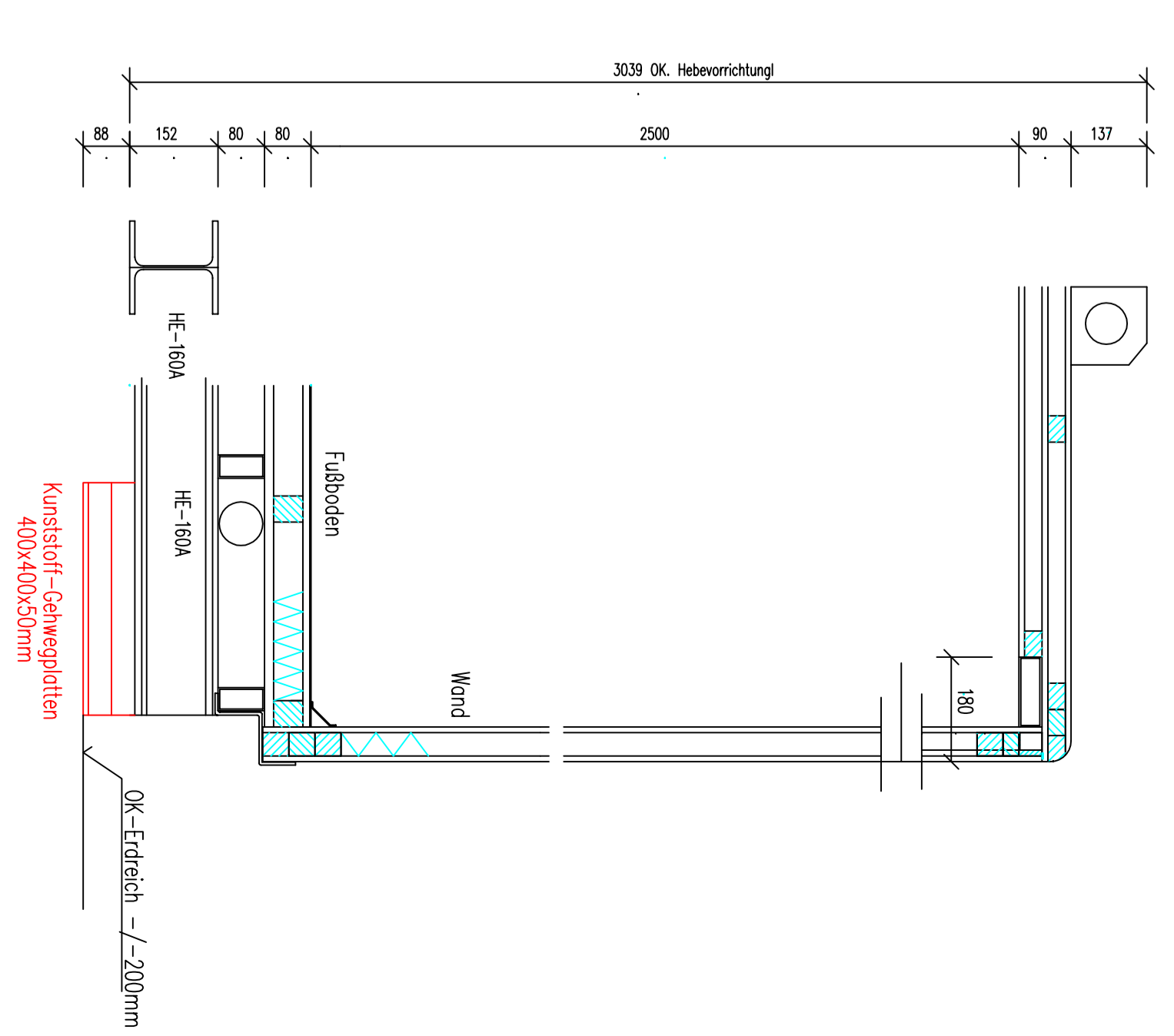
Schnitt A-A
