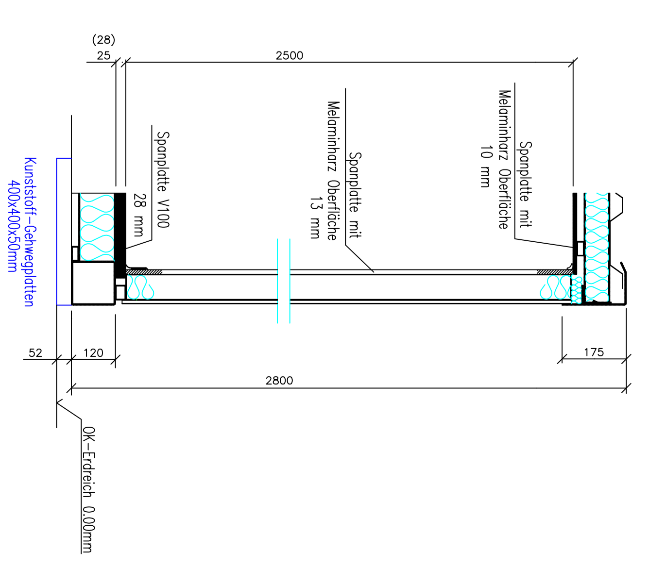
Schnitt B-B
